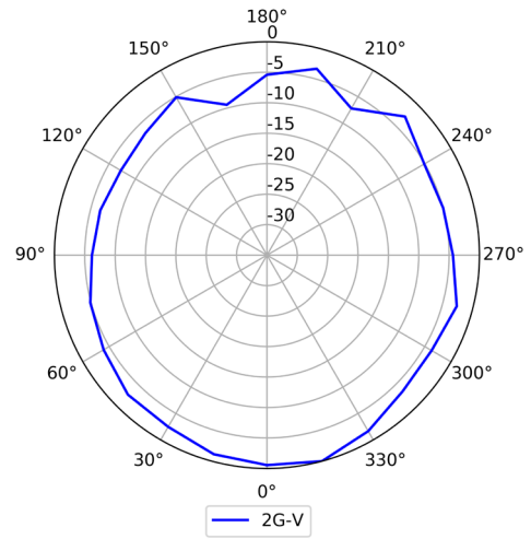
2.4G (Vertical)
