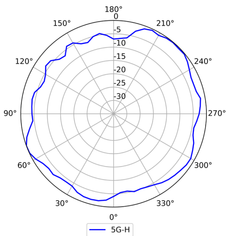
5G (Horizontal)
