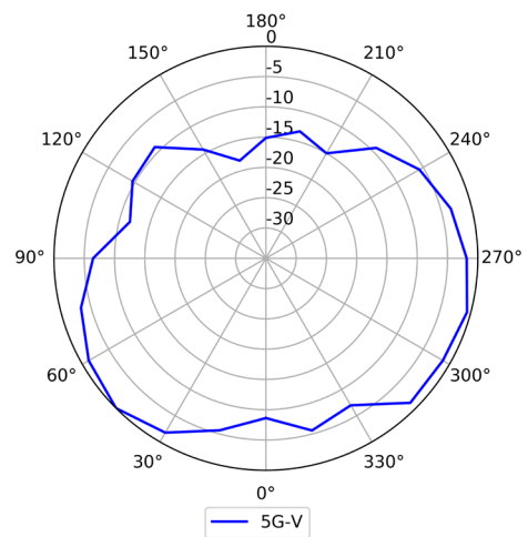
5G (Vertical)
